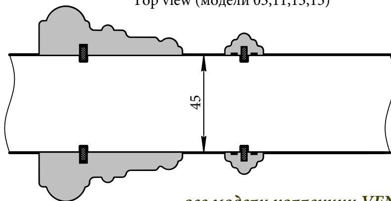
Top view (модели 03,11,13,15)
